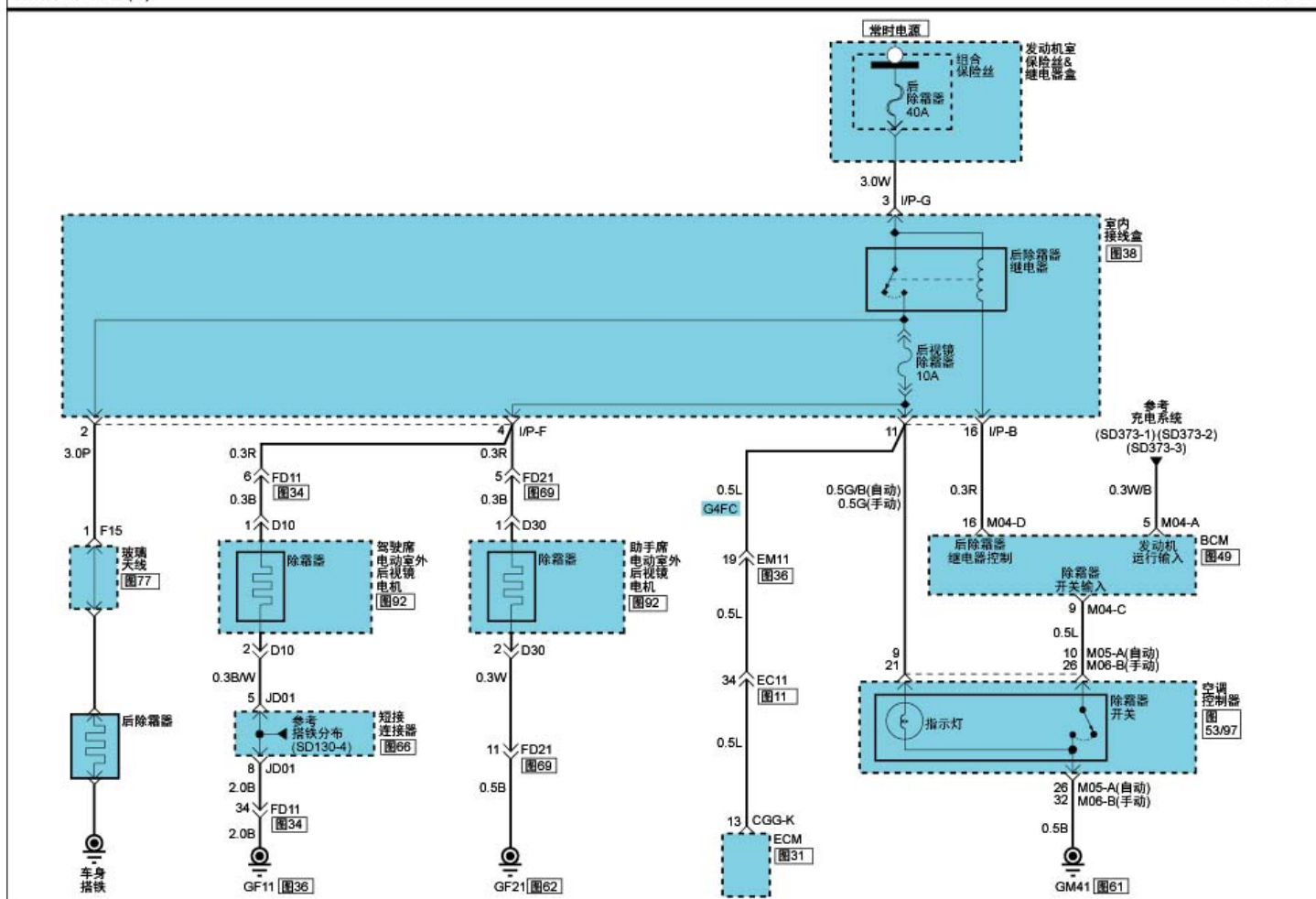
除霜器系统(1)
